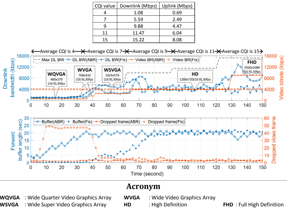
Figure A.18: Débit maximal mesuré pour chaque valeur de CQI et les résultats obtenus.
